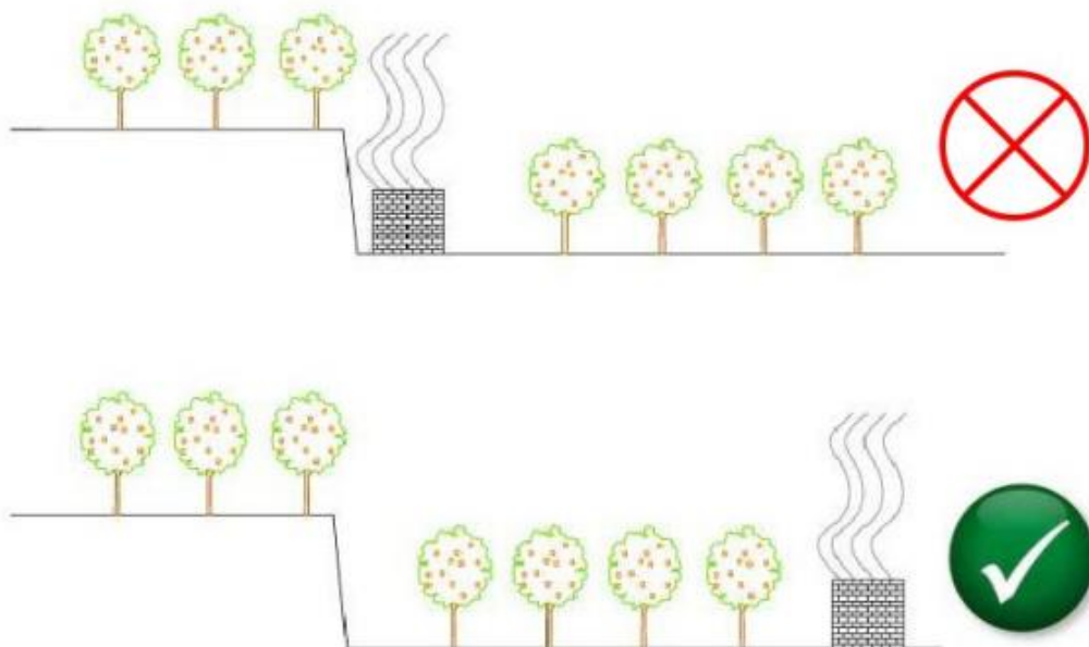
Ubicación idónea de un quemador agrícola dentro de una parcela abancalada. Fuente: Norma Técnica de Quemadores Agrícolas (PPIFD Polinyà del Xúquer).
