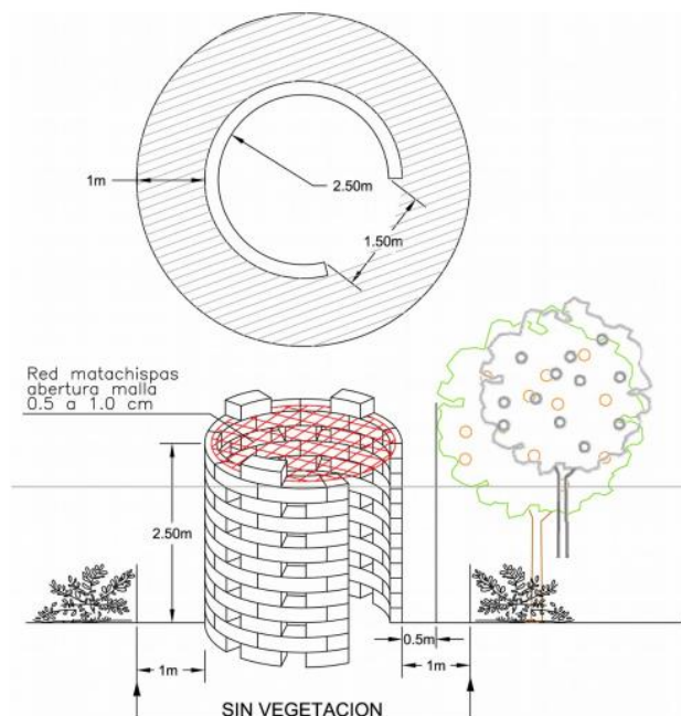
Planta y alzado de un quemador debidamente condicionado. Fuente: Norma Técnica de Quemadores Agrícolas (PPIFD Polinyà del Xúquer).
